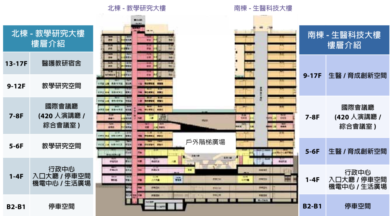
圖二：雙和校區樓層配置圖
