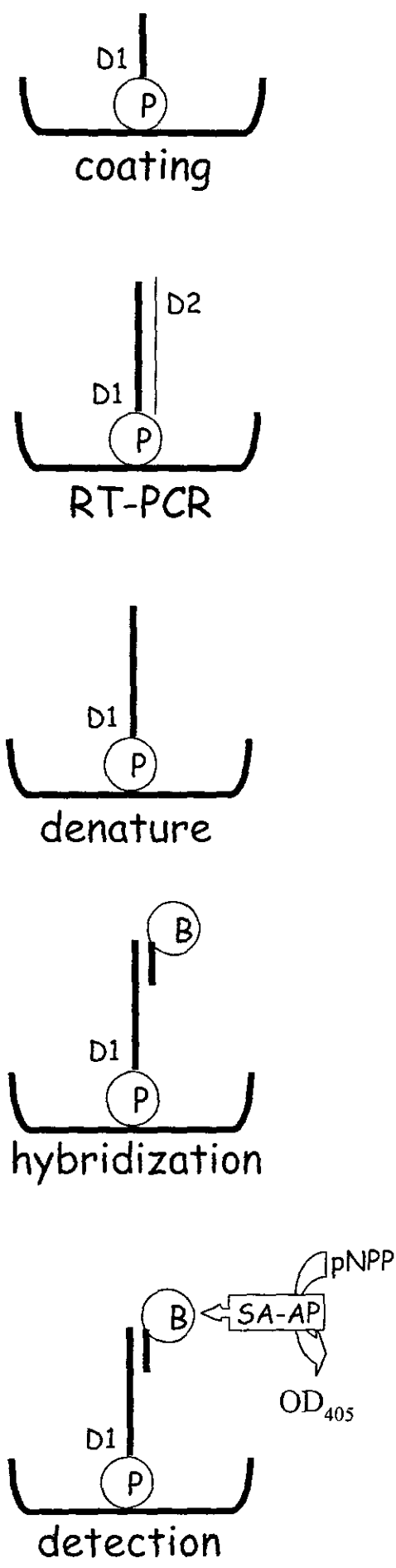
圖四 以5'端標示磷酸根之PCR引子D1塗佈之微量滴定盤，進行RT-PCR/ELISA的流程。呈色物質(biotin)標示於登革特異性探針引子之5'端。
