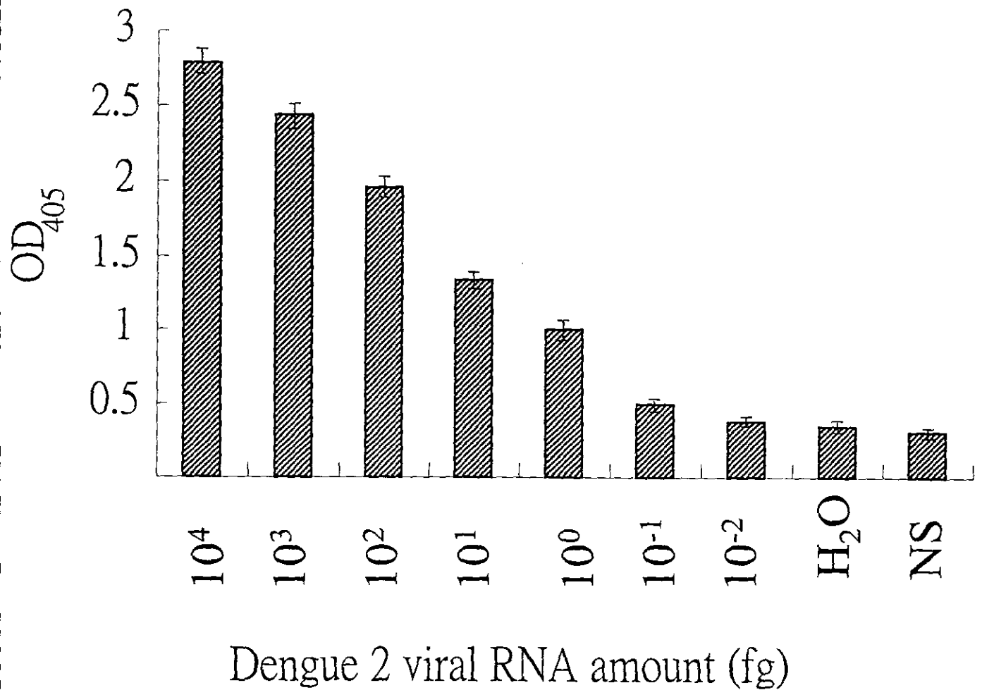
圖十：以 streptavidin coated plate based assay 檢測第二型登革病毒之靈敏度。病毒 RNA 以 fg 為單位，H 2 O 為 negative control，NS 為登革病毒陰性血清檢體。
