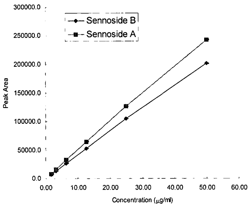
圖二、Sennosides A 及 B 之標準曲線。
