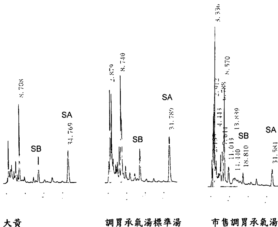
圖一、調胃承氣湯中 Sennosides A 及 B 指標成分之 HPLC 含量分析圖。 Sennoside B (SB)及 Sennoside A (SA) 滯留時間分別為 18.8, 34.5 分。
