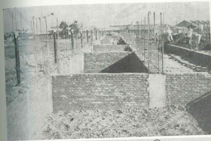
↓ 三層大廈第二幢基牆打竣
